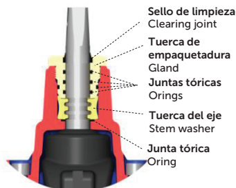
Válvulas de compuerta de cierre elástico de DN40 a DN200 Soft sealing gate valve DN40 up to DN200
